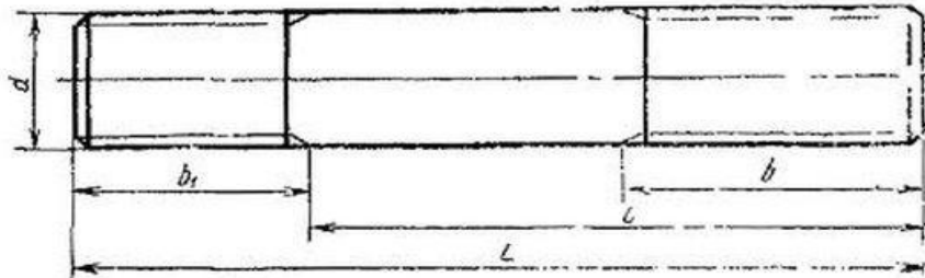
Шпилька для фланцевых соединений М20х95 А
