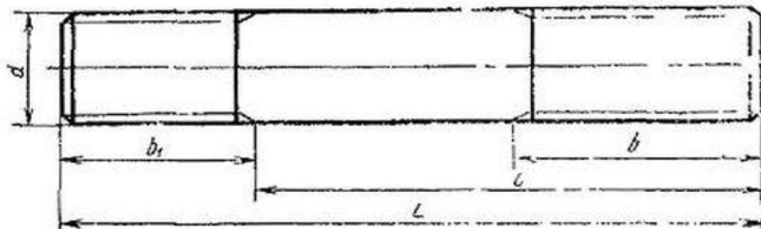
Шпилька для фланцевых соединений М30х220 А
