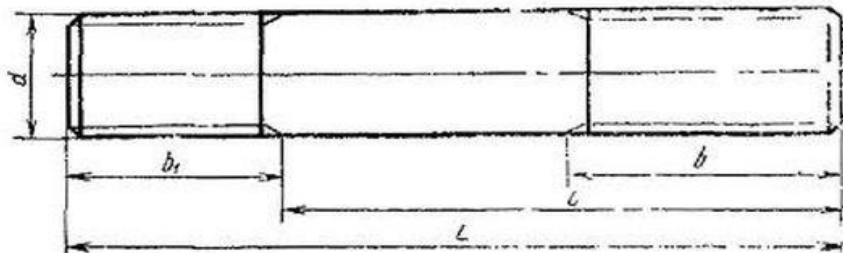
Шпилька для фланцевых соединений М36х370 А
