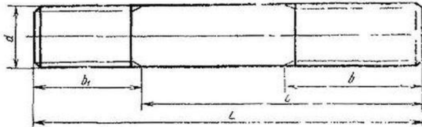
Шпилька для фланцевых соединений М42х300 А
